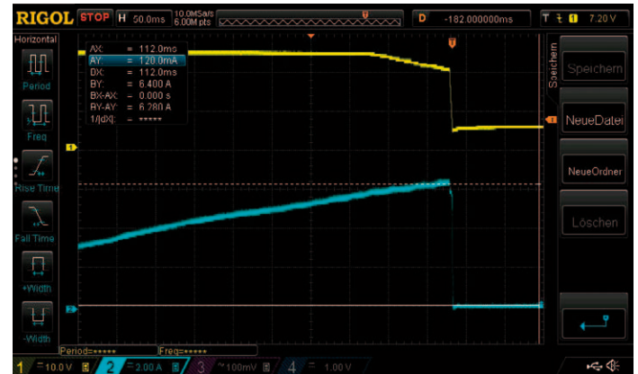
Bild 4: Überstromabschaltung (OCP) eines 24 V/115 W Netzteils (blau Strom, gelb Ausgangsspannung)
