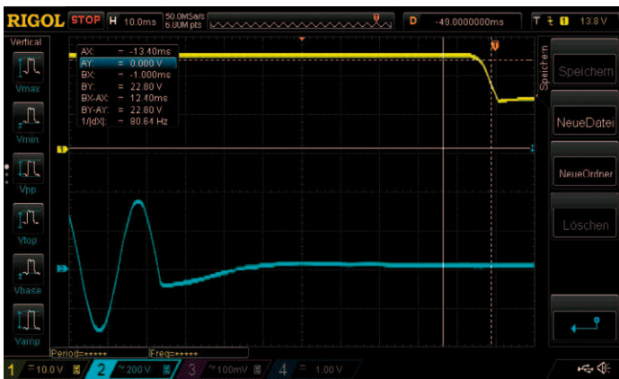
Bild 11: Hold-Up-Zeit an Netzteil Klasse A PFC mit 230V AC Eingang
