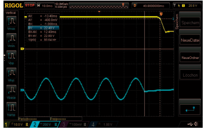
Bild 10: Hold-Up Zeit an Netzteil Klasse A PFC mit 110V AC Eingang
