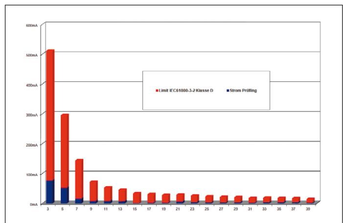
Bild 8: Harmonische Oberwellen PFC Klasse D (rot Limit, blau Messwert)
