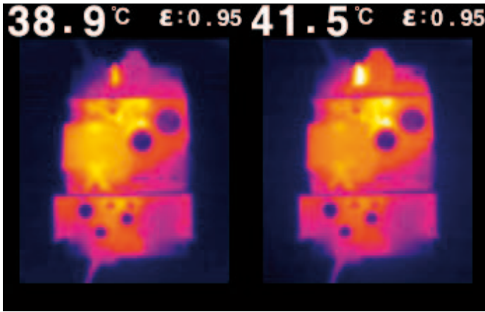
Bild 9: Schaltnetzteil an 230V AC (links) und 110V AC (rechts)
