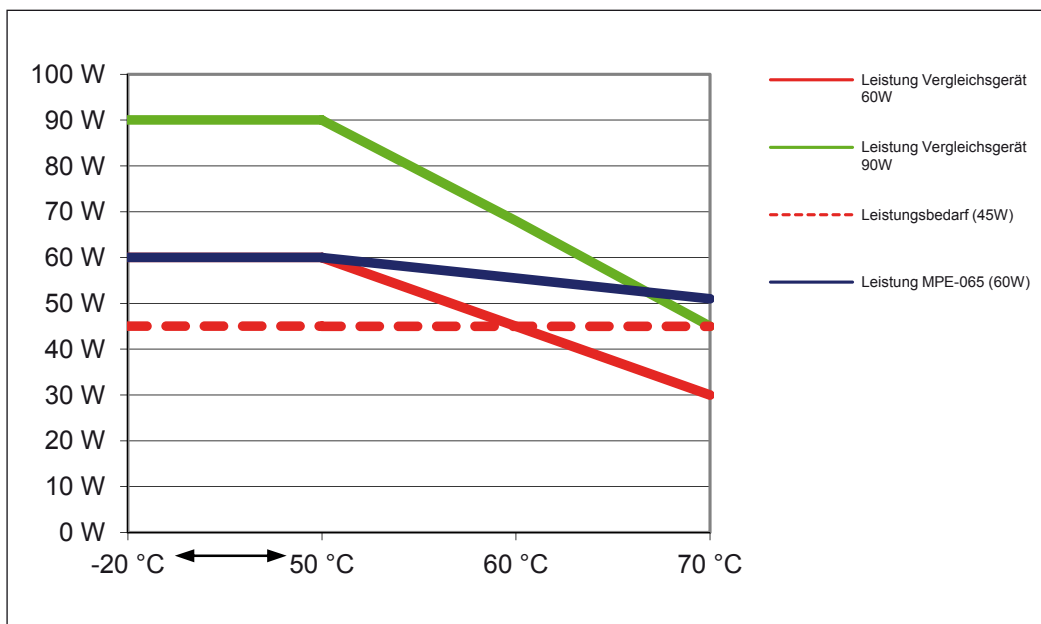
Bild 13: Vergleich Derating MPE-S065 zu Vergleichsgeräten
