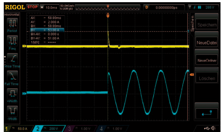
Bild 12: Messung Einschaltstrom
