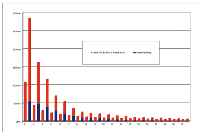
Bild 7: Harmonische Oberwellen PFC Klasse A (rot Limit, blau Messwert)
