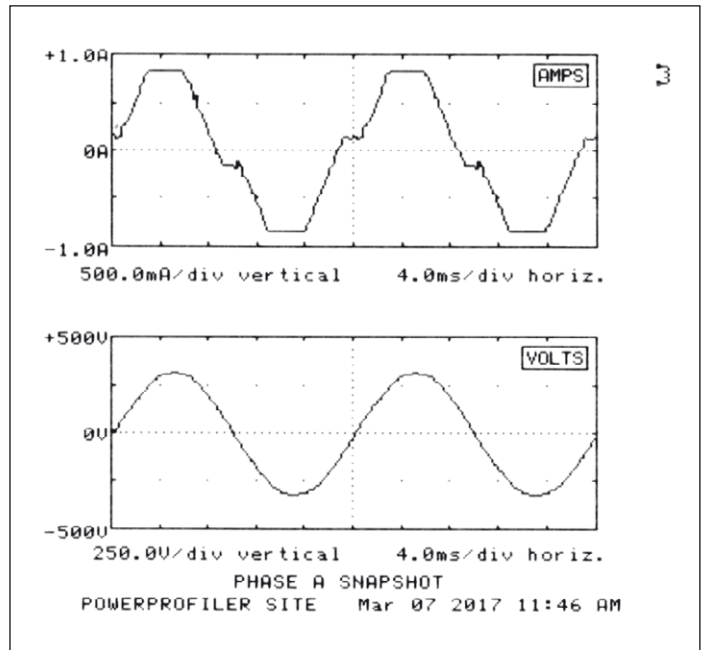
Bild 6: Stromverlauf Netzteil 120 W mit aktiver Klasse D PFC
