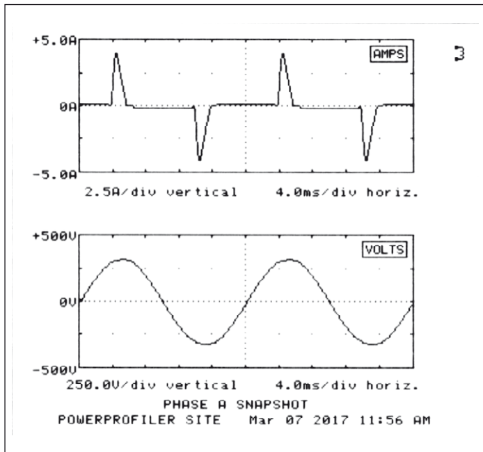
Bild 5: Stromverlauf Netzteil 120 W mit passiver Klasse A PFC
