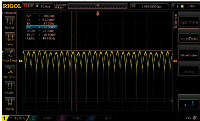
Bild 1: Messung mit Prüfspitze und Masseleitung
