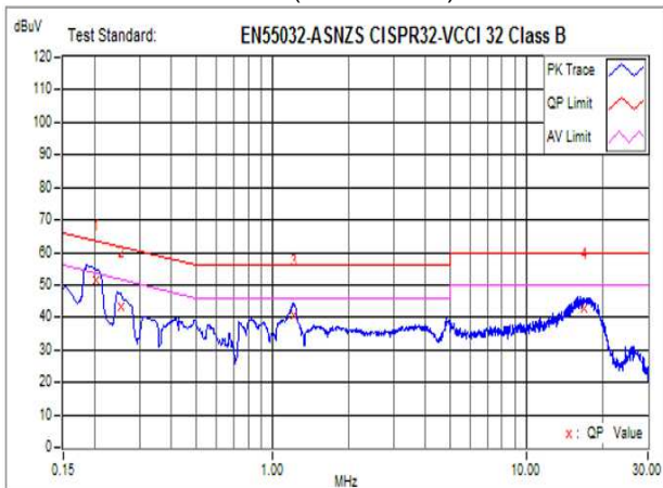
EMI: EN 55032 "B" (Conduction)
