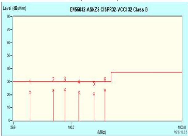
230Vac/max load
