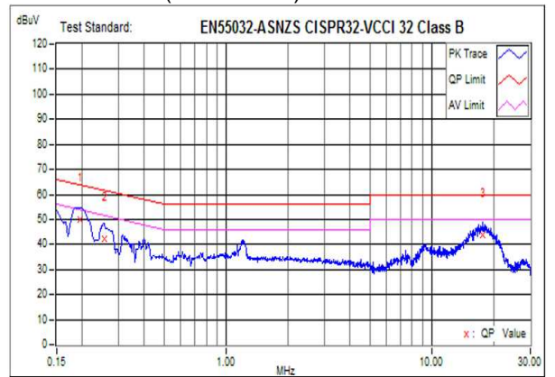
115Vac/max load
