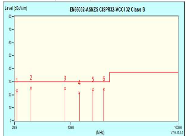
115Vac/max load
