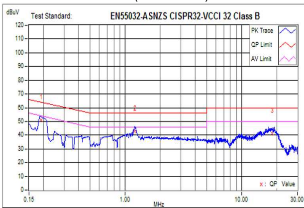
230Vac/max load
