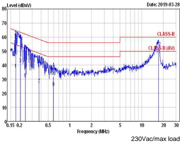
EMI: EN 55032 "B" (Conduction)
